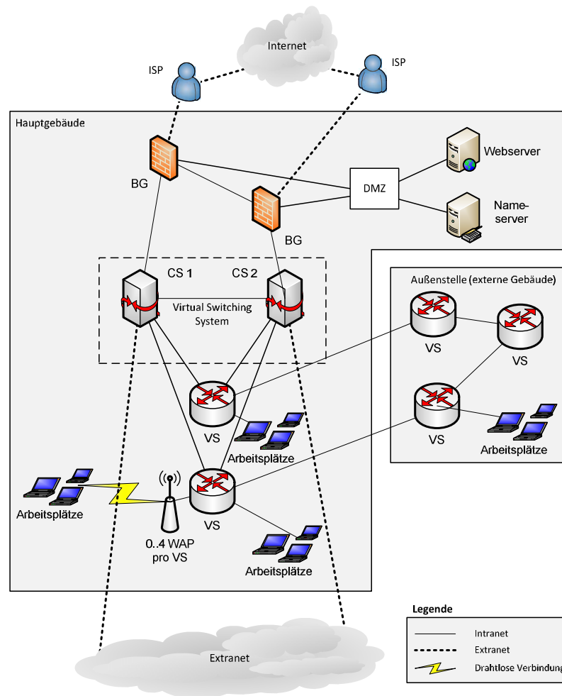
Abbildung 4: Netzwerk-Struktur eines Standorts [RaGP13]
