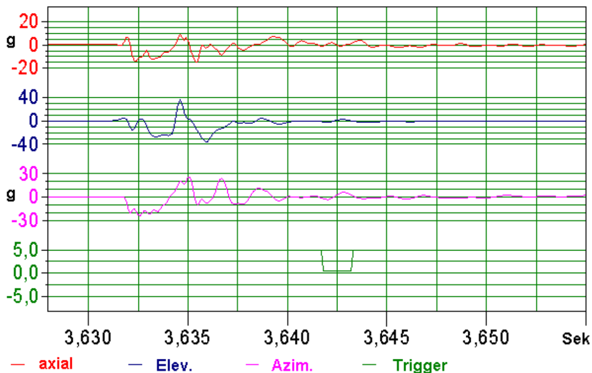
Abb. 4.24: Schwingungsdiagramme für Gewehr ANSCHÜTZ, Schuss Nr. 1, v_2 = 350.3m/s ; 19.07.2010 in Liegenstellung.
