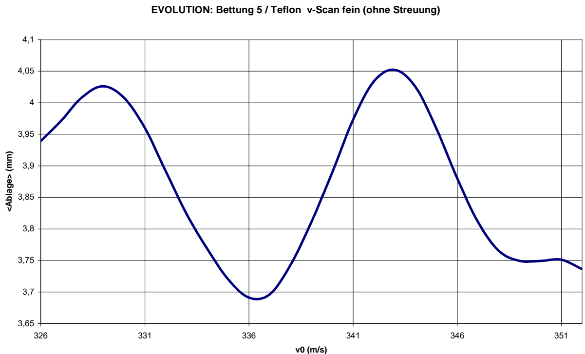
Abb. 5.32: „ v_0 -Scan“ fein für Versuchsgewehr EVOLUTION, Bettung 5/Teflon. Keine v_0 -Streuung. Die <Ablage>-Werte ergeben sich nur aus der Streuung der radialen Exzentrizität. Beachtung des Ordinatenmaßstabes!
