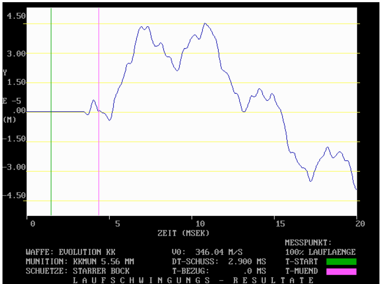
Abb. 5.8: Mit ROSSI gerechneter Zeitverlauf der Mündungsposition für das Versuchsgewehr EVOLUTION in der vertikalen Ebene bis 20 ms nach Schussbeginn. Der Schussbeginn ist der Zeitpunkt des Aufschlages des Schlagbolzens auf die Patrone. Die vertikale grüne Linie markiert den Bewegungsbeginn des Geschosses im Lauf. Die Zeit von 0 bis zur grünen Linie entspricht in ROSSI der Zeit, in der das Pulver in der Patrone bereits zu brennen beginnt, der Gasdruck aber noch nicht ausreicht, den Auszieh Widerstand des Geschosses aus der Patronenhülse zu überwinden. Die magentafarbene Linie markiert den Zeitpunkt des Geschosßdurchganges durch die Mündung.
