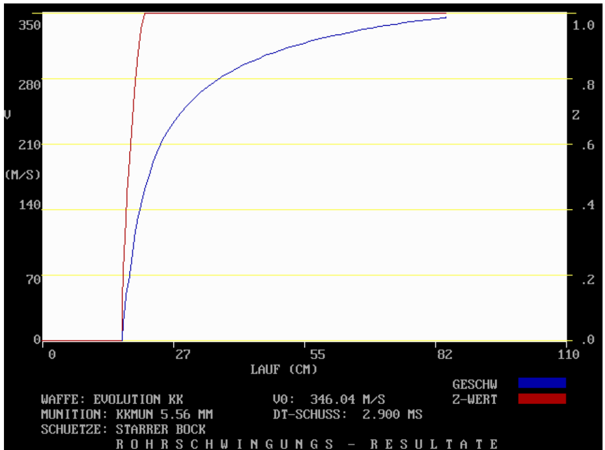
Abb. 5.28: Geschößgeschwindigkeit (blau) und Z-Wert (rot) in Abhängigkeit von der Geschößposition im Lauf. Anmerkung: Der Z-Wert ist das Verhältnis der Masse des verbrannten Pulvers zur ursprünglichen Pulvermasse. Der Pulverabbrand erfolgt hier sehr schnell.
