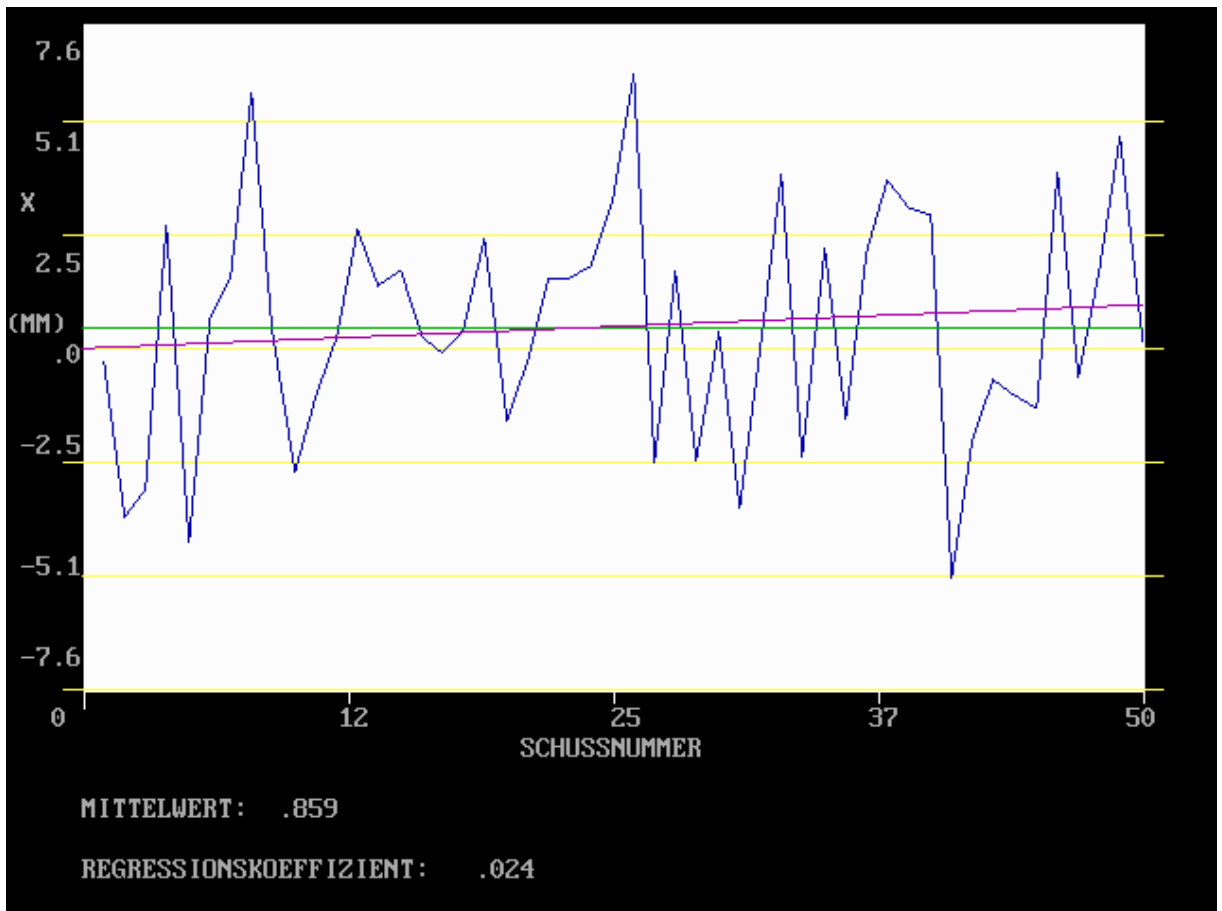
Abb. 4.26: Mit dem Programm ROST gerechnete Verteilung der x-Koordinaten einer 50 Schusserie. Die magentafarbene Linie ist die Trendlinie deren Anstieg der gesuchte Regressionskoeffizient ist. Die grüne waagrechte Linie markiert nur den Mittelwert über 50 Schuss der x-Koordinatenwerte.
