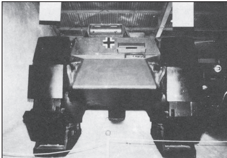
von vorne, Sechsschitz und Turm mit 2 MG Bild: Waffen Revue
