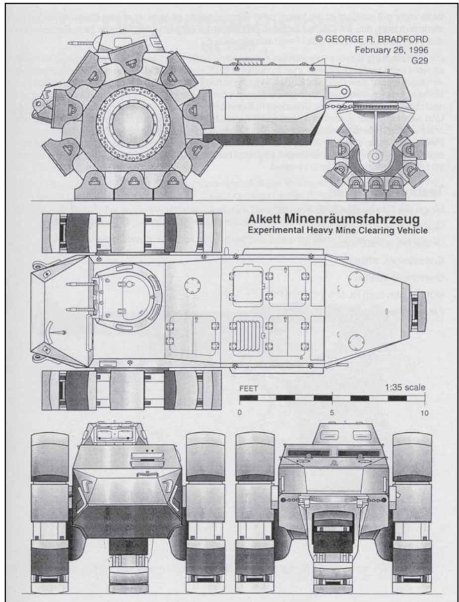
Alkett Minenräumfahrzeug
