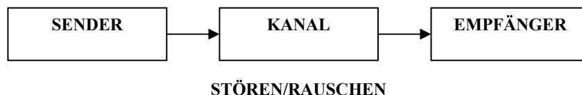
Abbildung 2: Sender-Empfänger Modell
