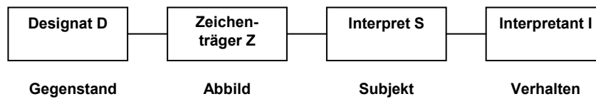
Abbildung 3: Semiose
