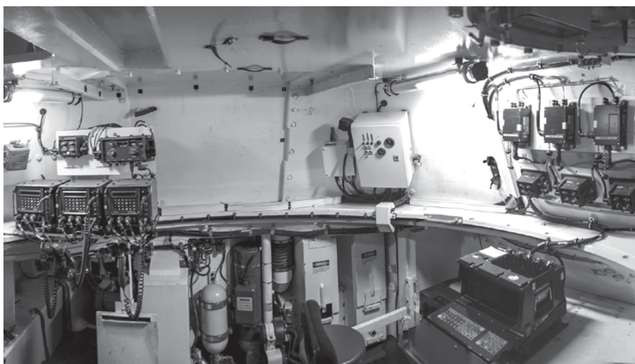
◀ Kampfraum des Rechenstellenpanzers mit elektronischem Artillerie- und Feuerleitsystem.
